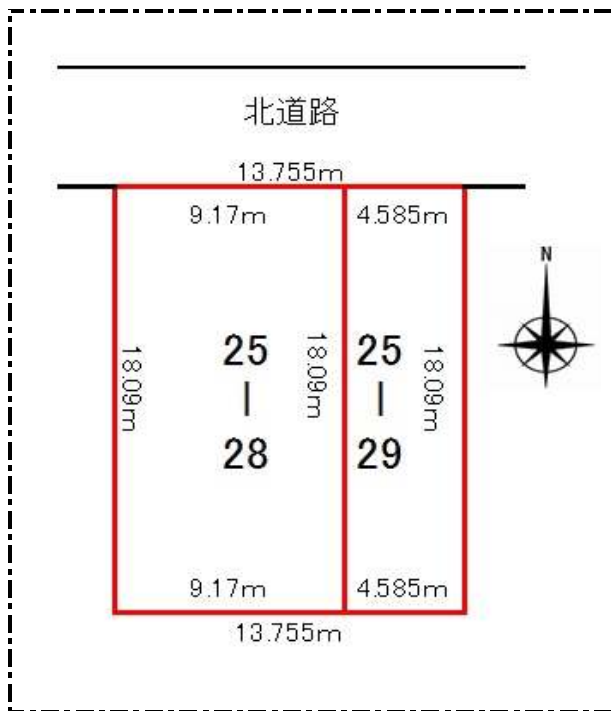
【 土地寸法図 】
